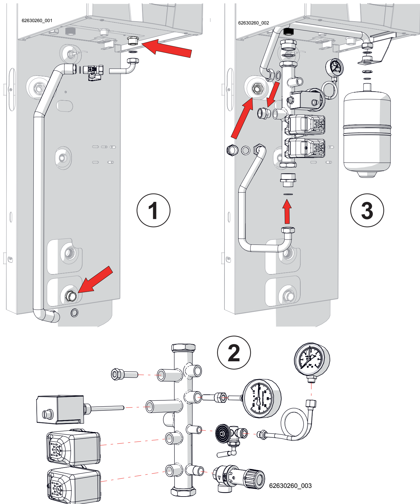
Figure 5-6 - Phases d'installation des tuyaux AGUADENS 37 (suite page suivante)
