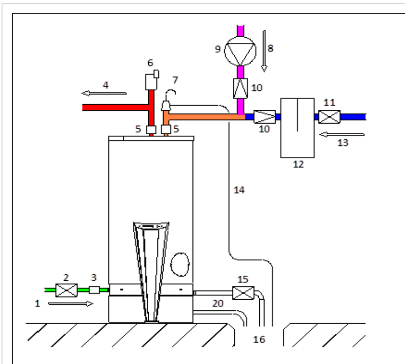
Fig. -6a schéma de principe, 1 accumulateur
