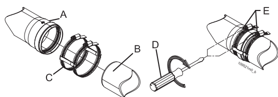
Figure 14-4 - Fixation des conduits d'évacuation et d'aspiration
