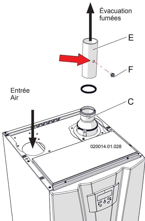
Figure 14-2 - Installation du système dédoublé
