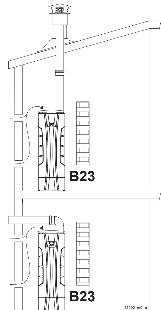
Figure 14-1 - Systèmes d'évacuation/d'aspiration
