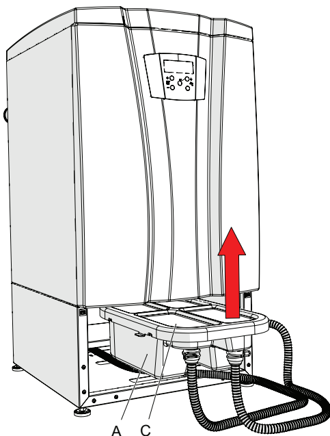
Figure 18-9 - Démontage et ouverture de la boîte de neutralisation de la condensation
