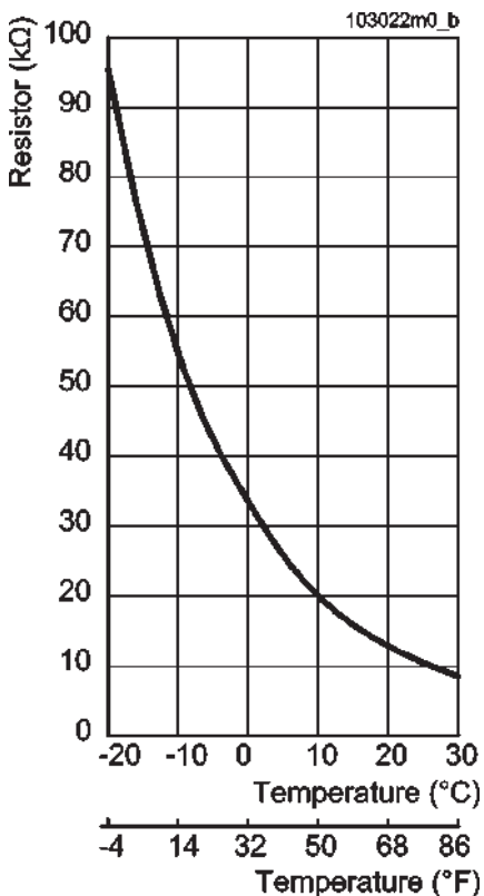
Figure 18-14 - Courbe du capteur température extérieure
