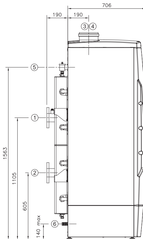
Vue latérale
