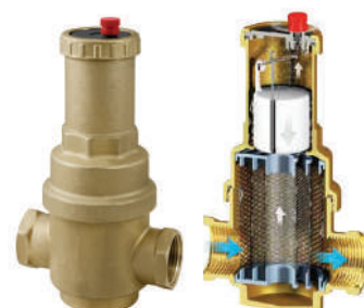
Séparateur d'air
