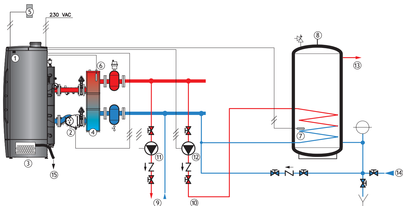
Schéma MYDENS 60 T - 70 T - 100 T - 115 T - 140 T
