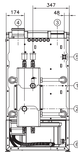
Vue postérieure
