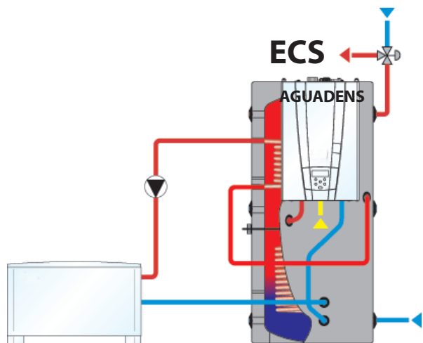
Connexion avec un ventilo convecteur
