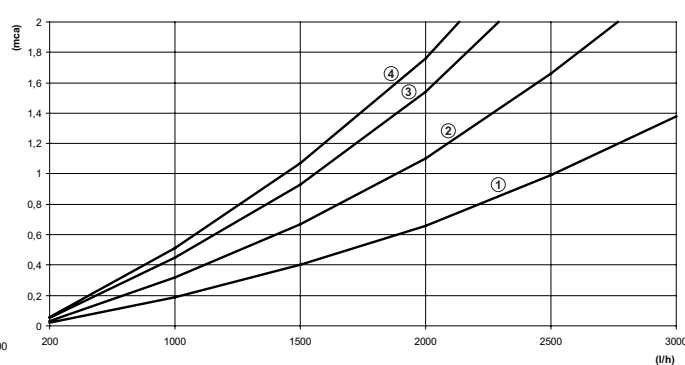
Serpentin supérieur + inférieur en série
