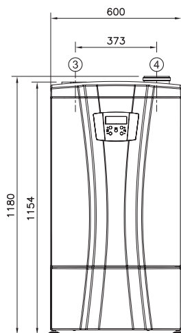
Vue frontale
