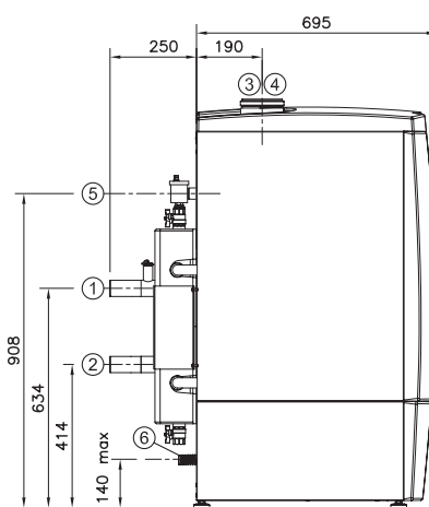
Vue latérale
