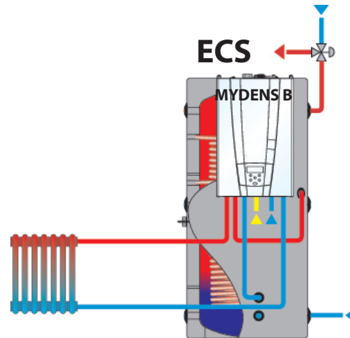
Connexion avec une chaudière MYDENS B
