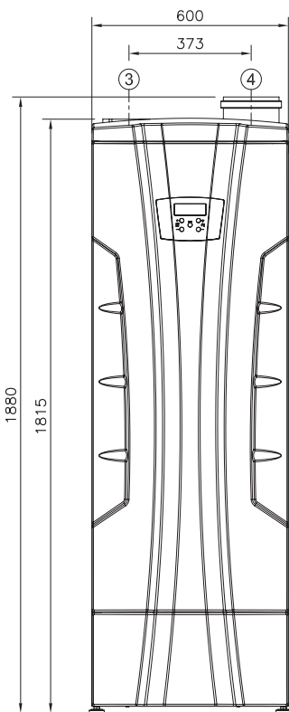
Vue frontale
