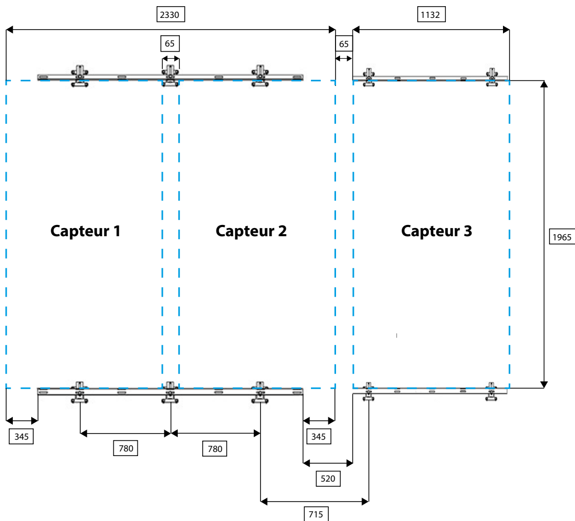
Illustration 4 : Distances entre les trous (mm)
