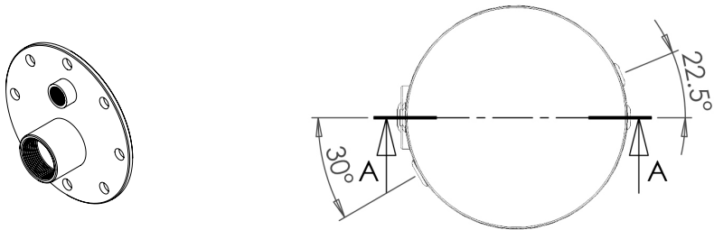
Bride pour résistance et sonde
